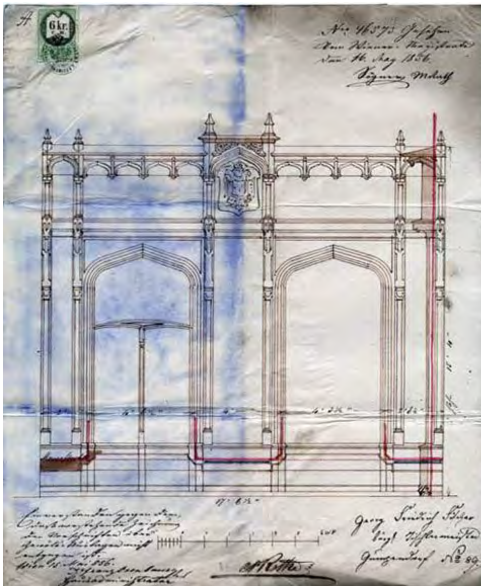
Abbildung 198: Fassadenentwurf von Georg Friedrich Fischer (1856)
